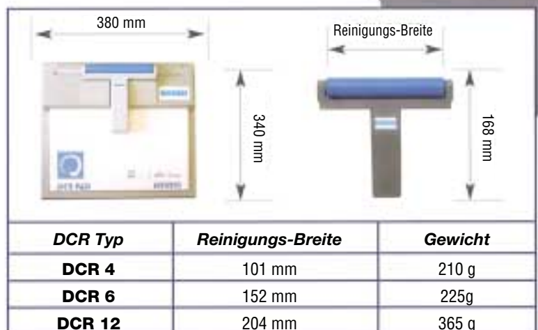
DCR-Roller-Reinigung
