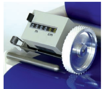
Folien Schneidgerät Modell B, Rollenbreite 109 cm oder 140 cm Folienablängvorrichtung mit einem Längsschneidklingenhalter und einem Meterzähler
